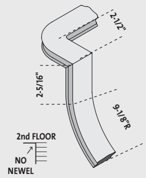
SP104 1 Riser 1/4 Turn No Cap - Right SP104-40C - PC
